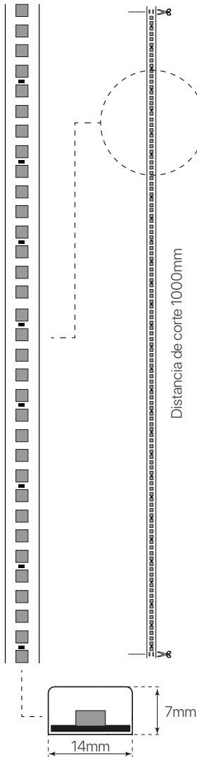
Rectificador 6A 230V no incluido
